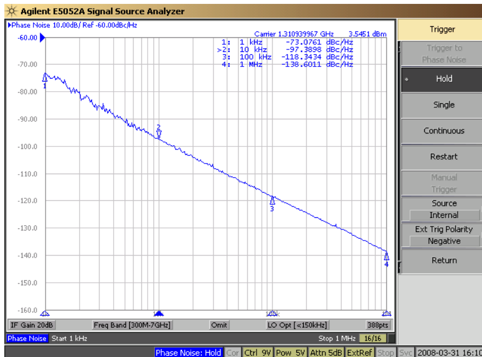
No.4 位相雑音 9.0v
