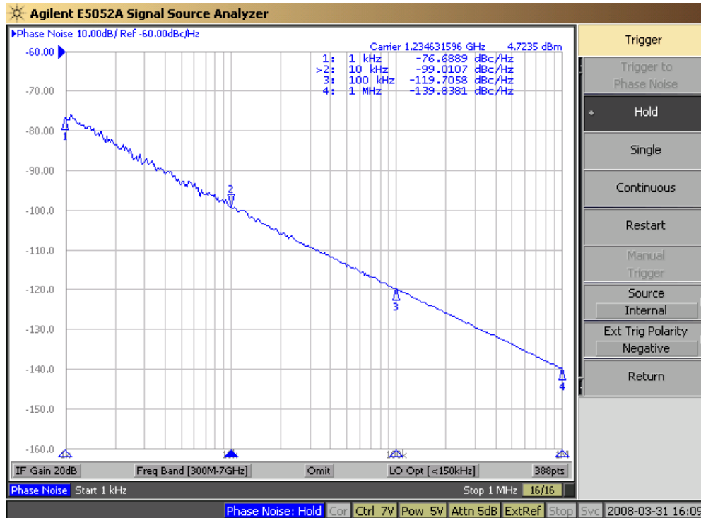
No.3 位相雑音 7.0v
